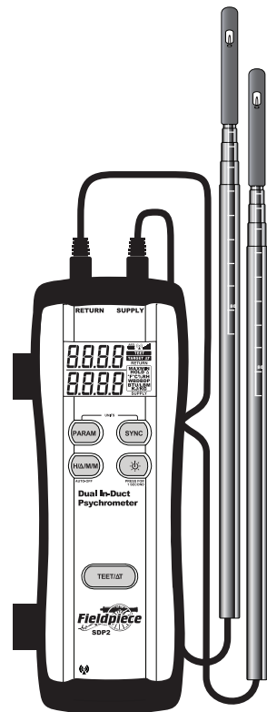
Modelo SDP2 Psicrómetro dual para conductos
